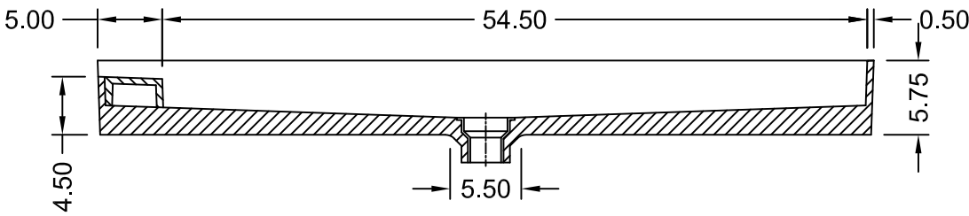
SECTION A-A
